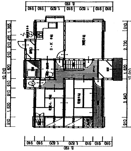
1階平面詳細図 S=1/100
